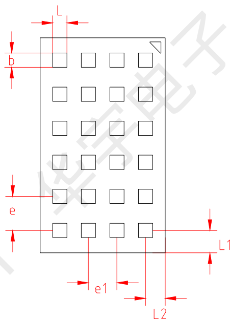
BOTTOM VIEW 背视图
